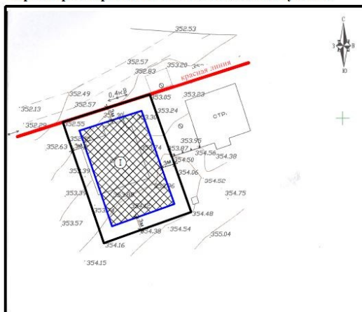
Чертеж градостроительного плана земельного участка
